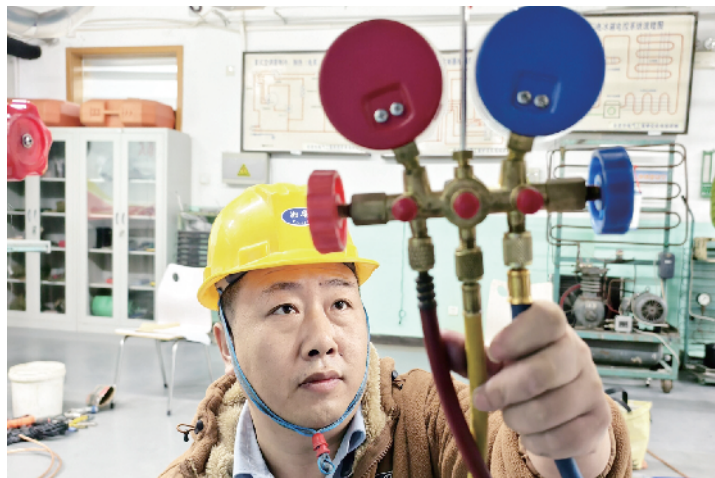
制冷设备更换干燥过滤器操作考核中，选手观察氟利昂数值
