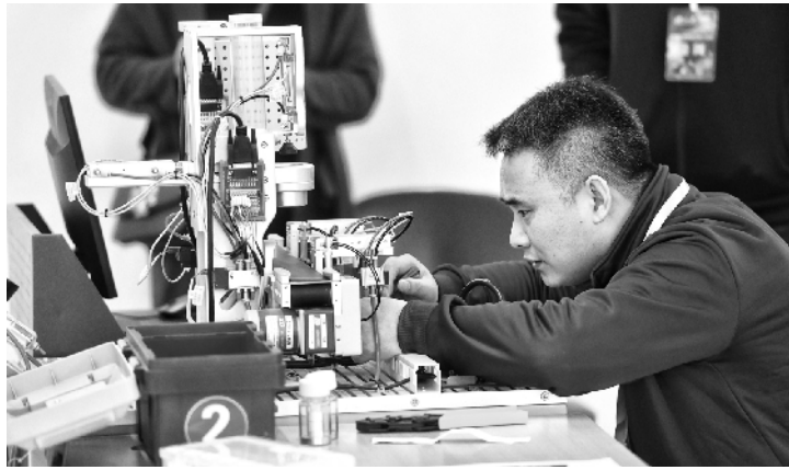
单元电气控制系统装调、搬运单元六轴机械臂应用编程、入库单元触摸屏组态与编程共四个项目的考核。 北京工业职业技术学院机电工程学院机电一体化技术专业负责人李林琛担任本场比赛的专家组组长。他坦言，此次选树活动是对选手综合能力的考核。比赛依据国家职业分类大典对自动控制工程技术人员定义，结合生产实际，选取典型工作任务，以智能产线为竞赛平台，考核参赛选手的电气设计、程序编写、安装调试、系统集成和职业素养等综合能力。
