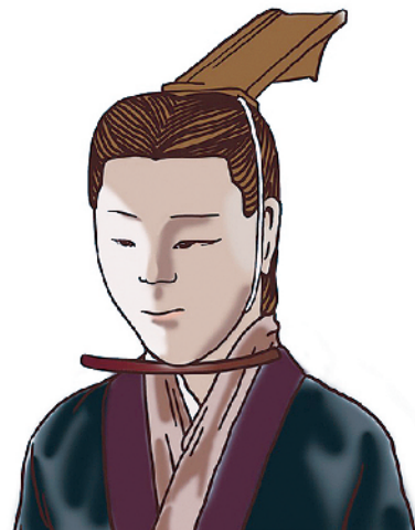
图3：刘氏冠
