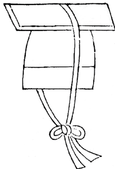
图4：樊哙冠
