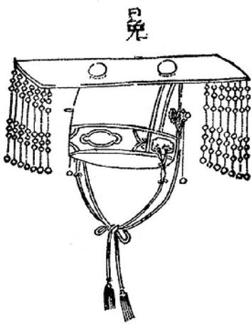
图1：七旒冕
