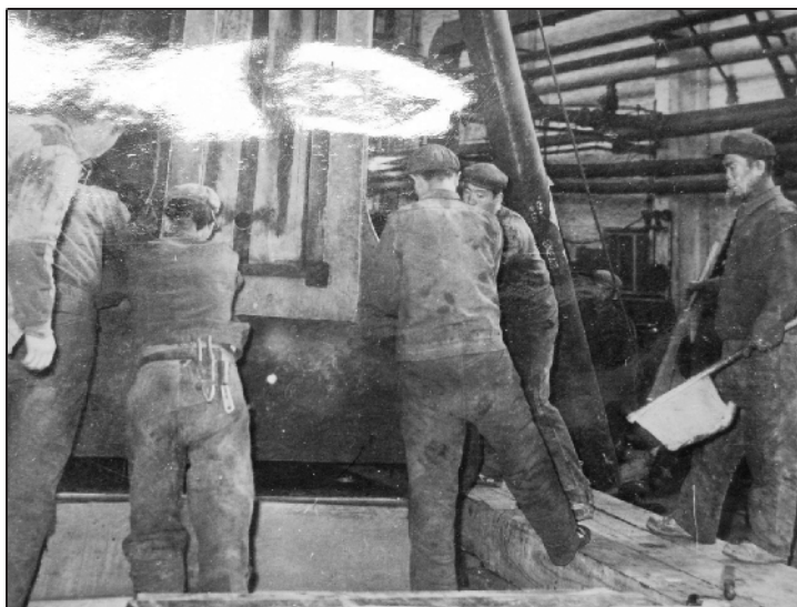
1964年10月，田恒仁正在内蒙古第一机械厂210车间现场指挥安装16吨锻锤的140吨锤砧。图中，田恒仁右手握着小红旗，嘴里吹着哨子，正在现场指挥。
